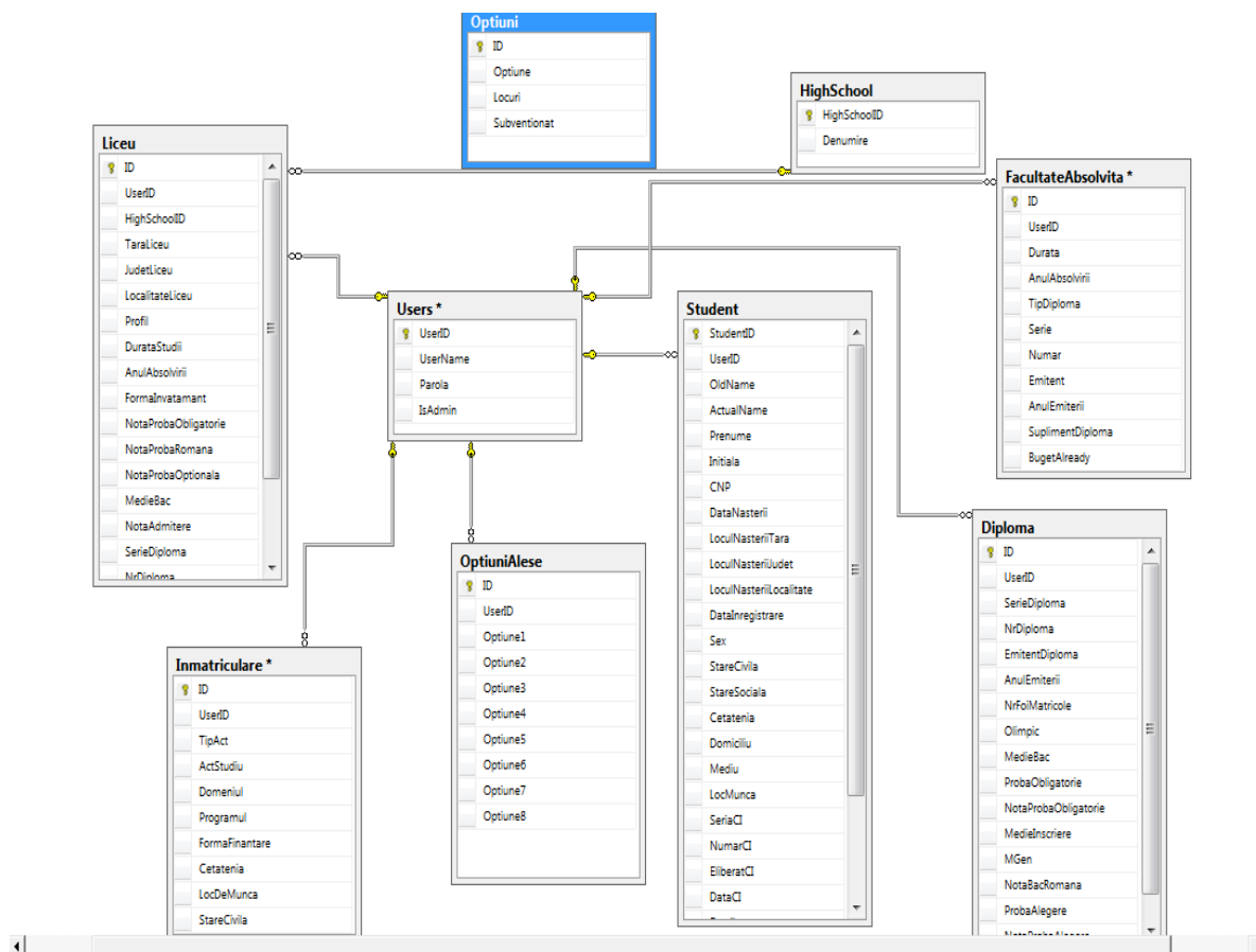
Fig.4. The database schema
